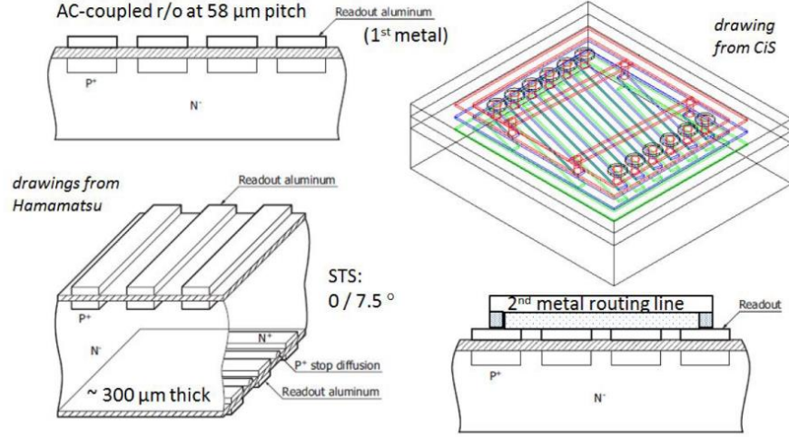
Şekil 2.6: CiS ve Hamamatsu dedektörlerinin üç boyutlu gösterimleri.
