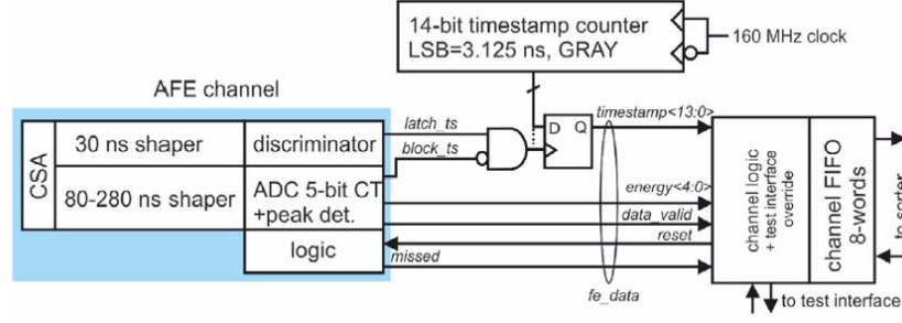
Şekil 2.19: Sinyal mekanizması.
