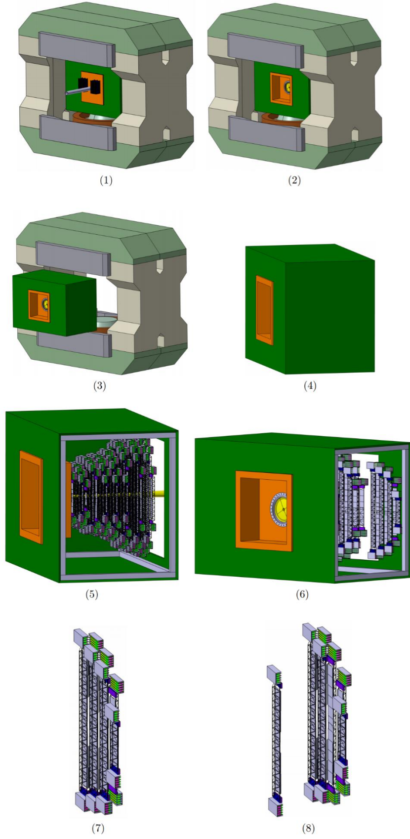
Şekil 2.4: Silikon izleme sisteminin dipol magnet içindeki görünümü ve iç parçaları [23].
