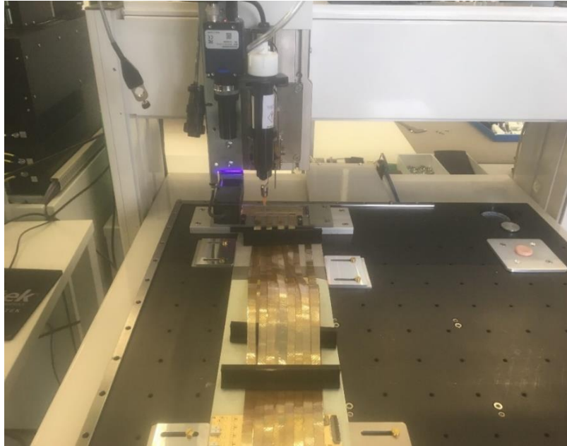
Şekil 3.24: Glop-top işlemi.
