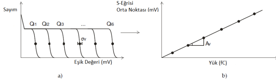
Şekil 3.14: (a) Birkaç s-eğrisi (b) Kazanç karakteristiği.
