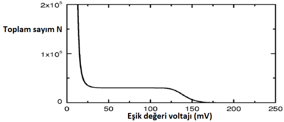
Şekil 3.12: Eşik seviyesine bağlı olarak ayırmıcadaki toplam sayım sayısı.
