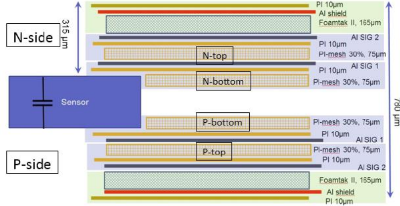
Şekil 2.15: Bir CBM modülü için mikrokabloların katmanları [43].
