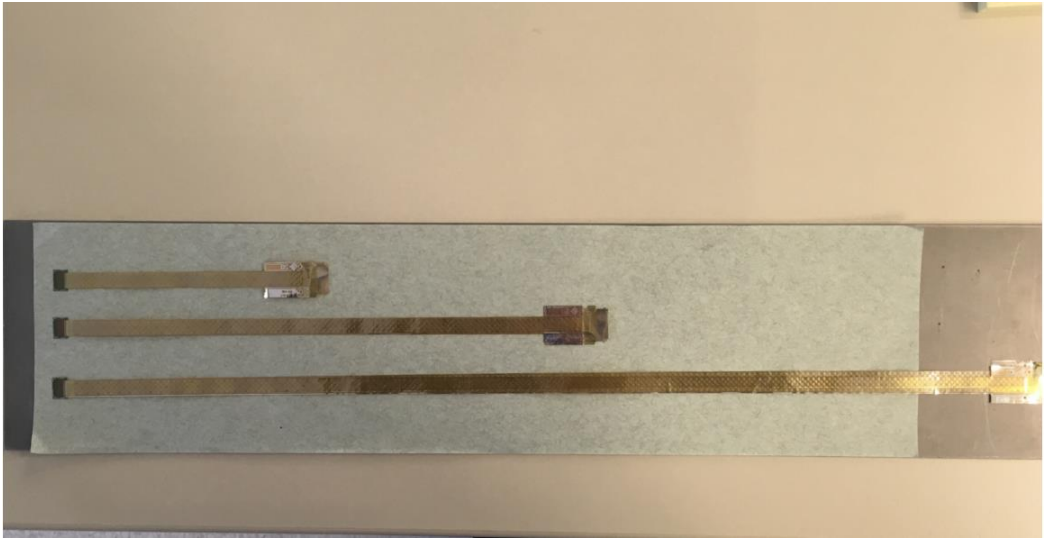
Şekil 4.7: Üç farklı mikro kablo uzunluğuna sahip çipler.
