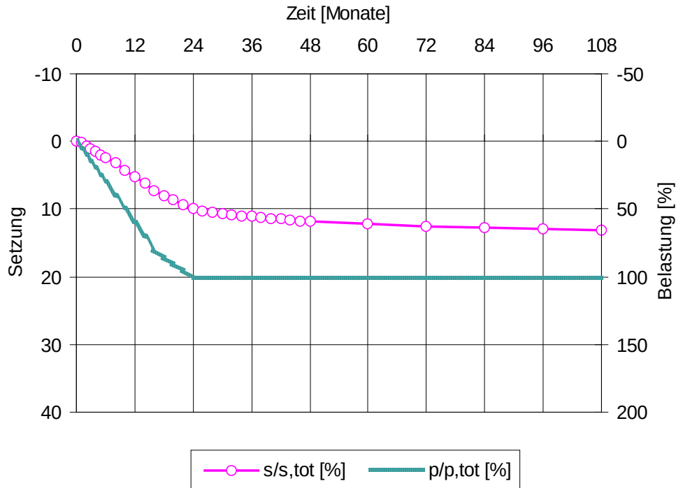
Bild 7.8 Zeit-Setzung eines Gebäudes
