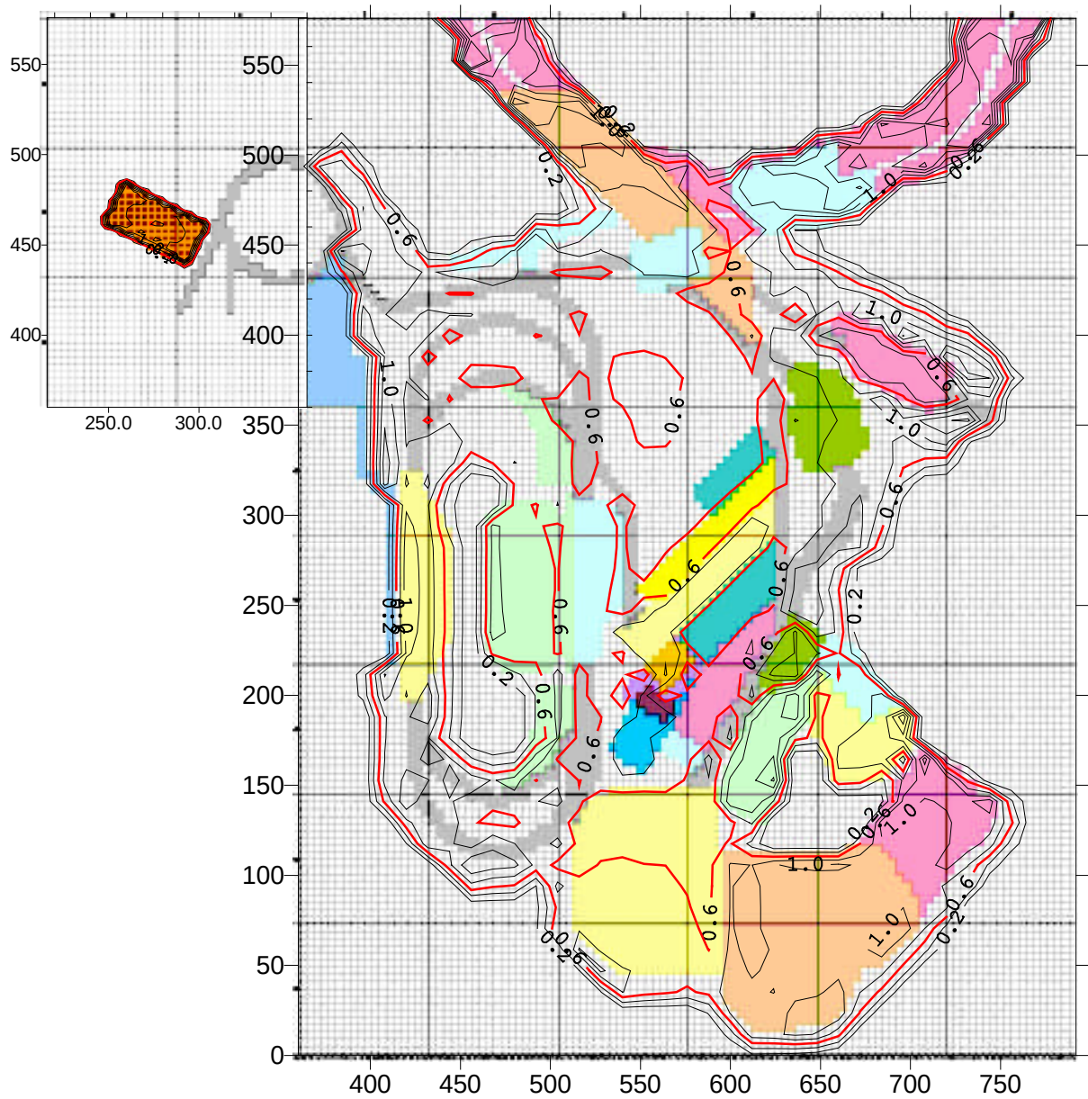
Bild 7.4: mittlere Bettungsmodulverteilung k_s [MN/m 3 ]
