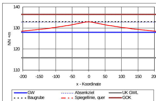
Bild 9.6: Auffülltrichter orthogonal zur Trasse
