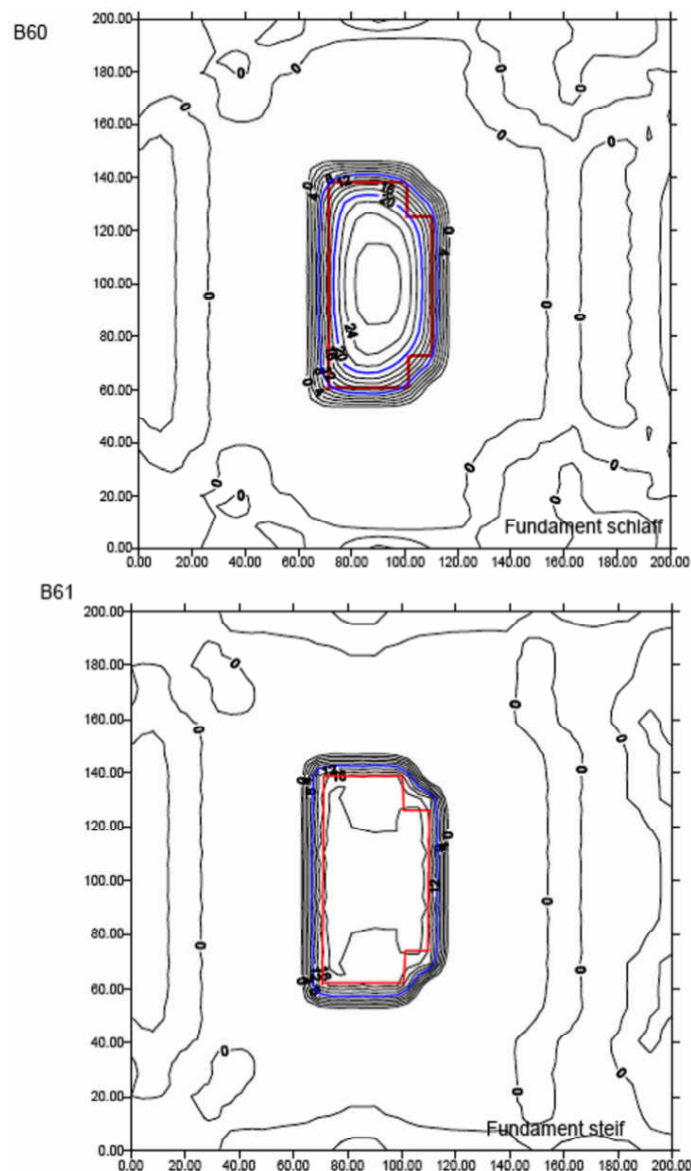
Bild 7.11: Einfluss der Biegesteifigkeit auf die Setzung
