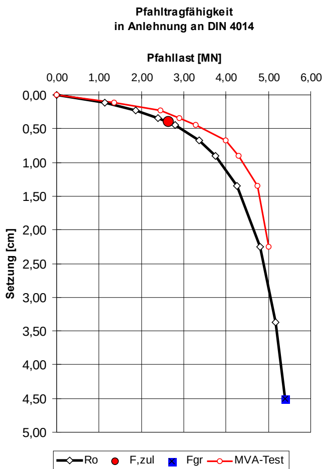
Bild 6.4: Last-Setzungsdiagramm Vergleichspfahl / Messung - Berechnung
