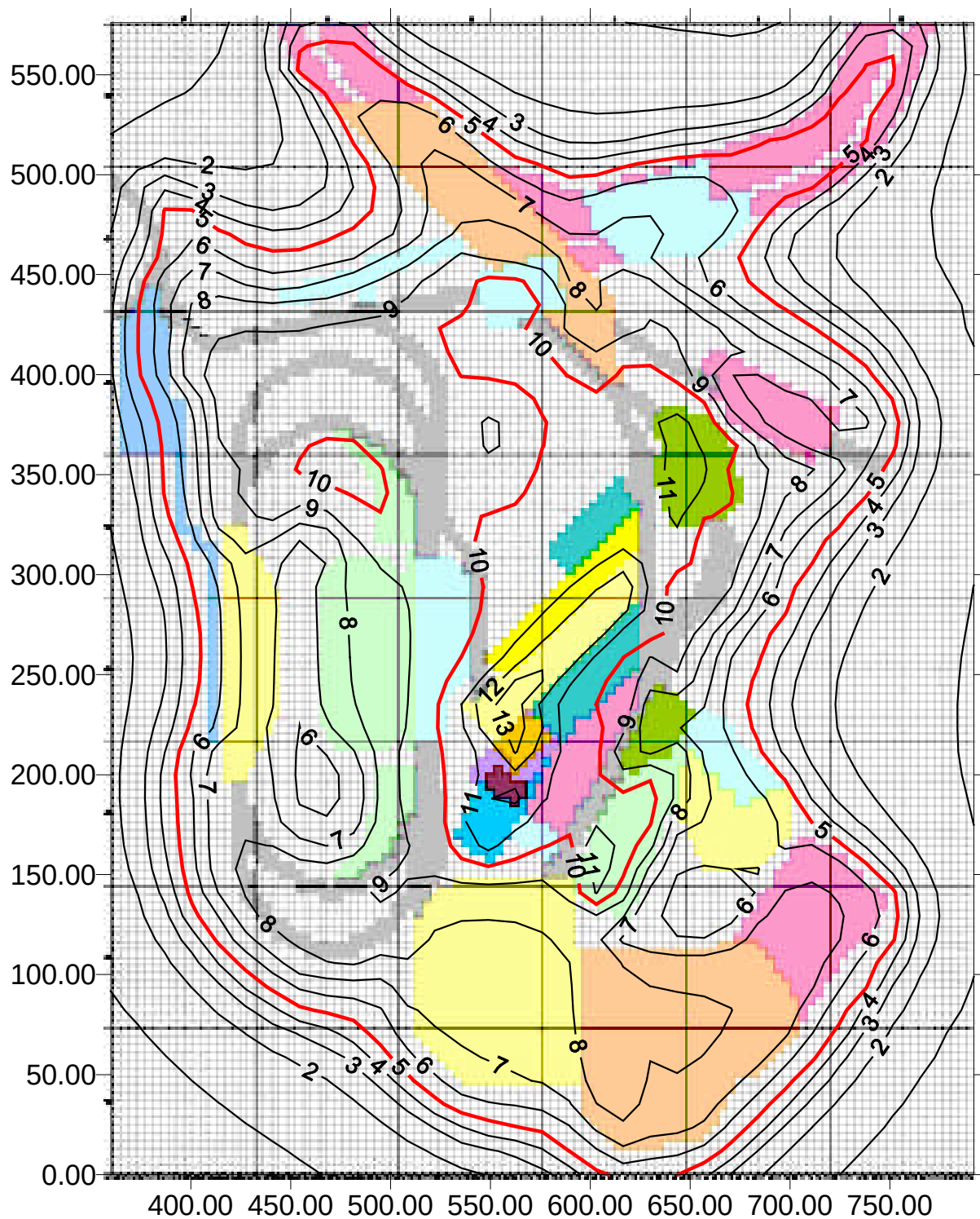
Bild 8.5 „optimale“ reduzierte Setzung mit ca. 2500 Pfählen
