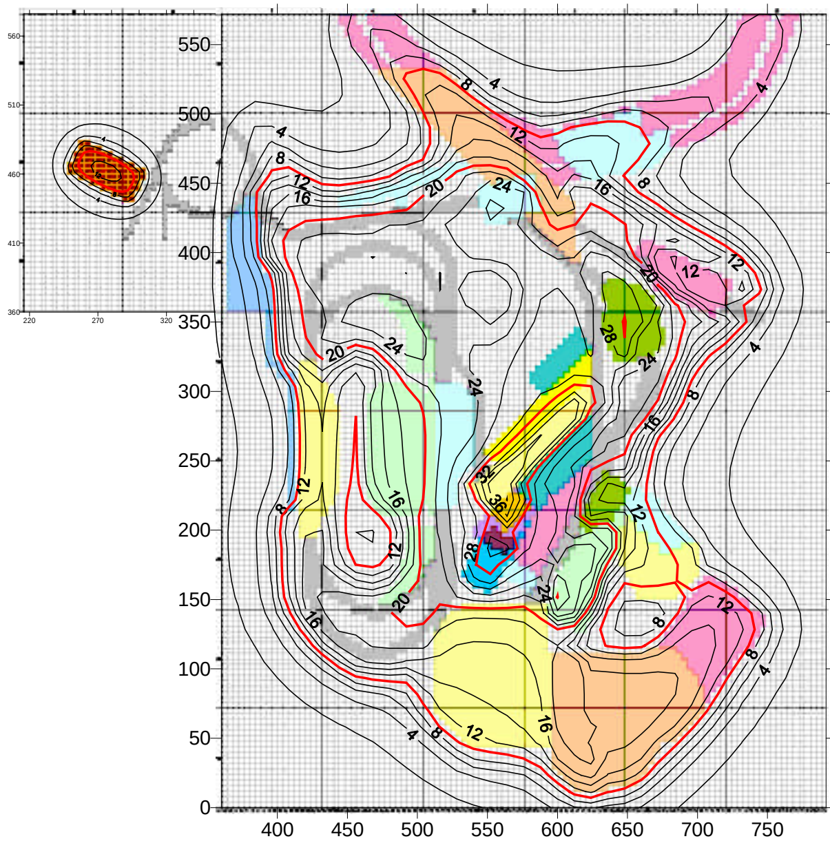
Bild 7.3: „wahrscheinliche“ Gesamtsetzungen
