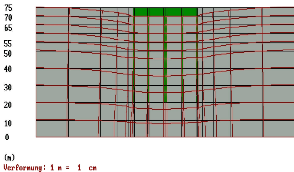
Verformtes Netz mit 50 m langen Pfählen s = 5 cm
