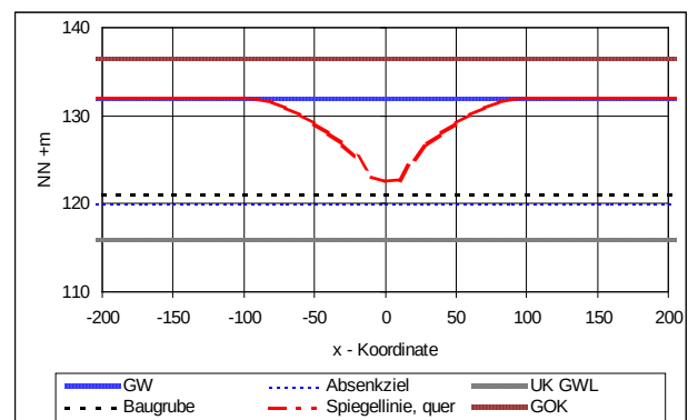
Bild 9.5 Absenktrichter orthogonal zur Trasse bei Versickerungsbrunnen in 100 m seitlichem Abstand
