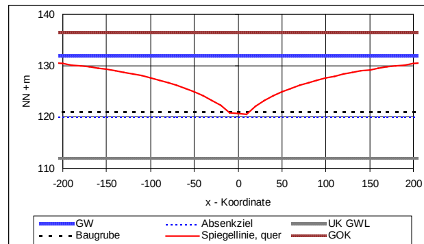
Bild 9.4: Absenktrichter orthogonal zur Trasse
