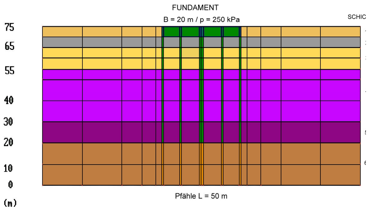
Bild 8.1 FE-Netz
