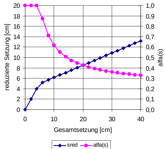
Bild 8.4: Setzungsreduktion
