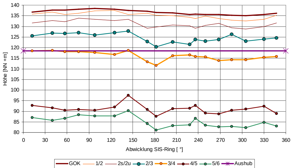
Bild 9.7: Lage des SIS-Tunnels
