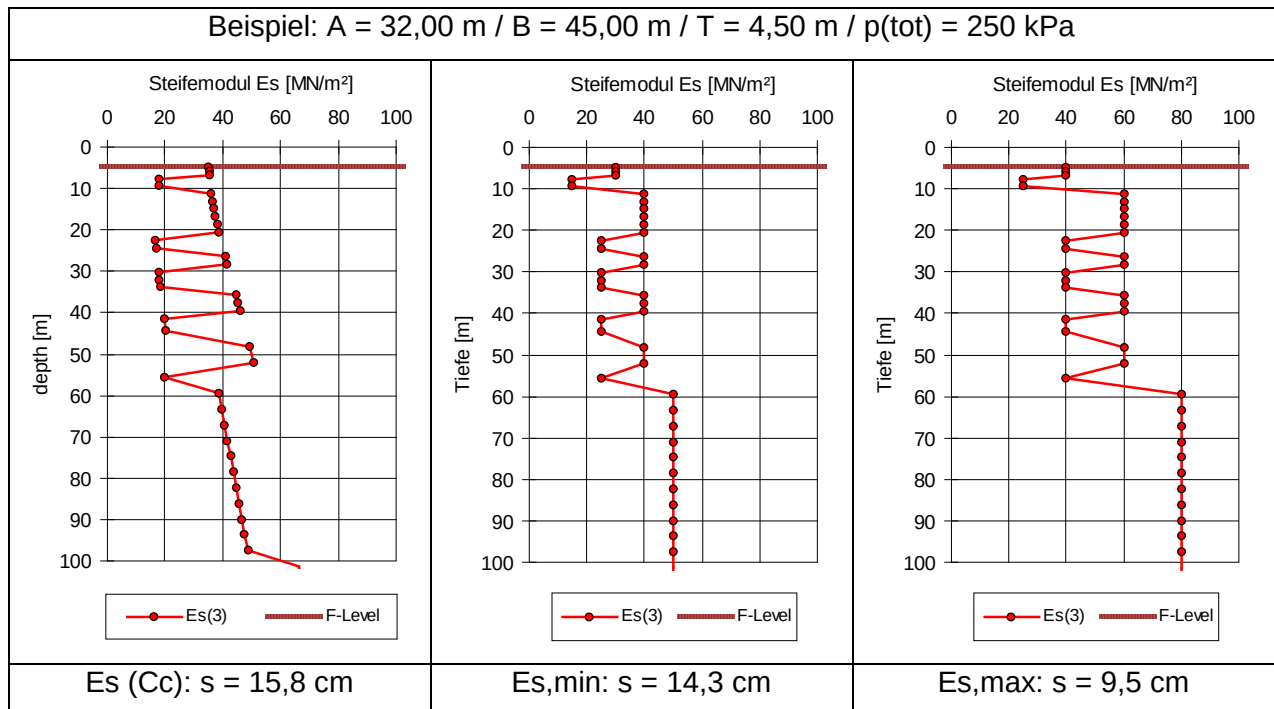
Bild 7.5: Verlauf des Steifemoduls nach der Tiefe
