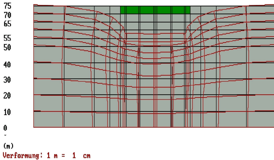
Verformtes Netz ohne Pfähle s = 16 cm
