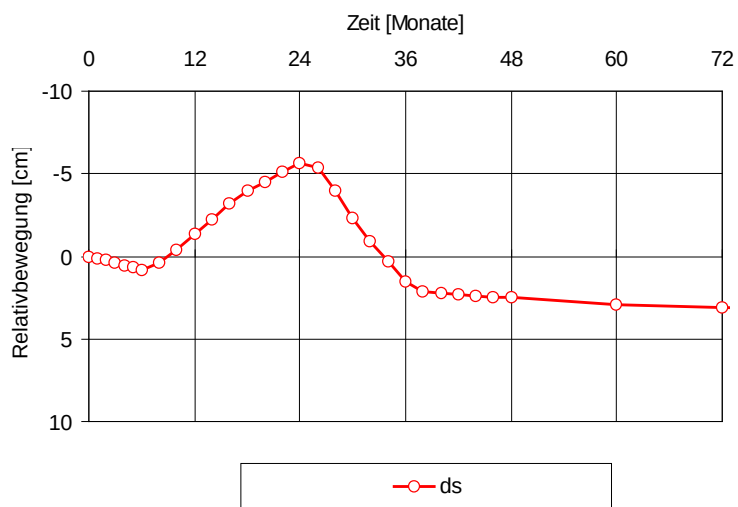
Bild 7.9: Setzungsablauf Beispiel 2
