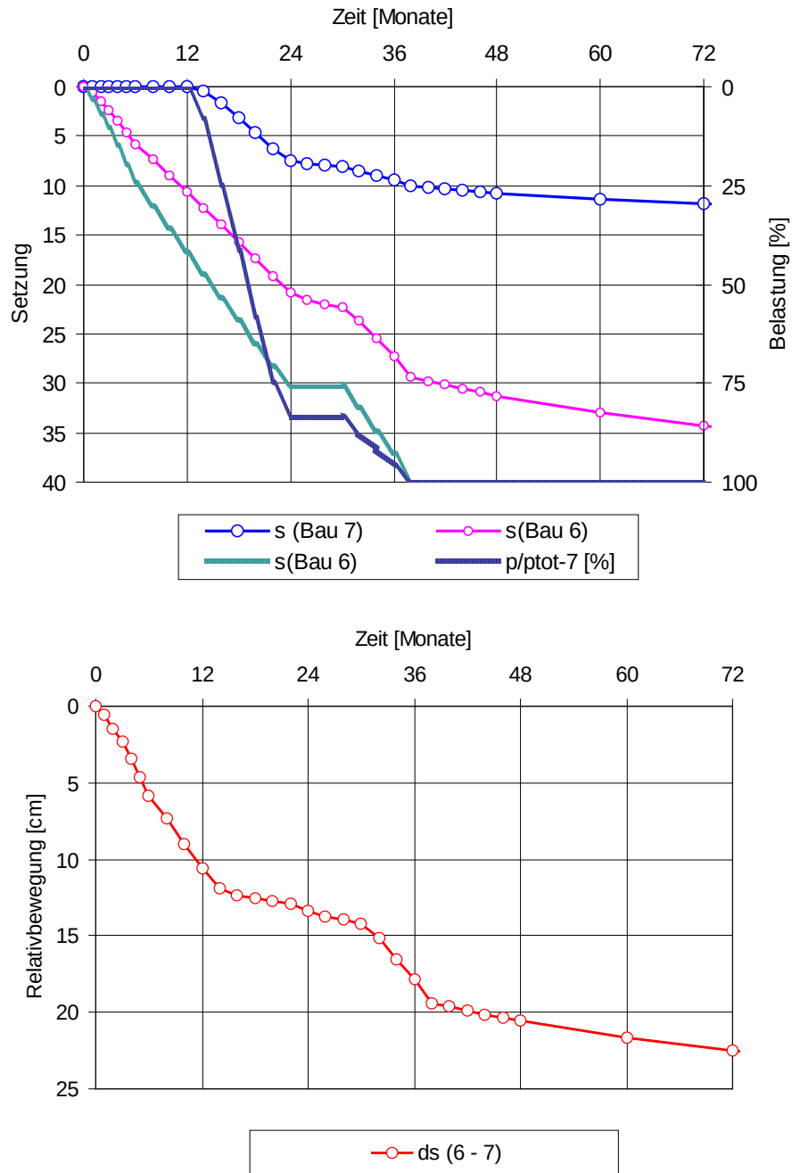
Bild 7.10: Setzungsablauf Beispiel 3
