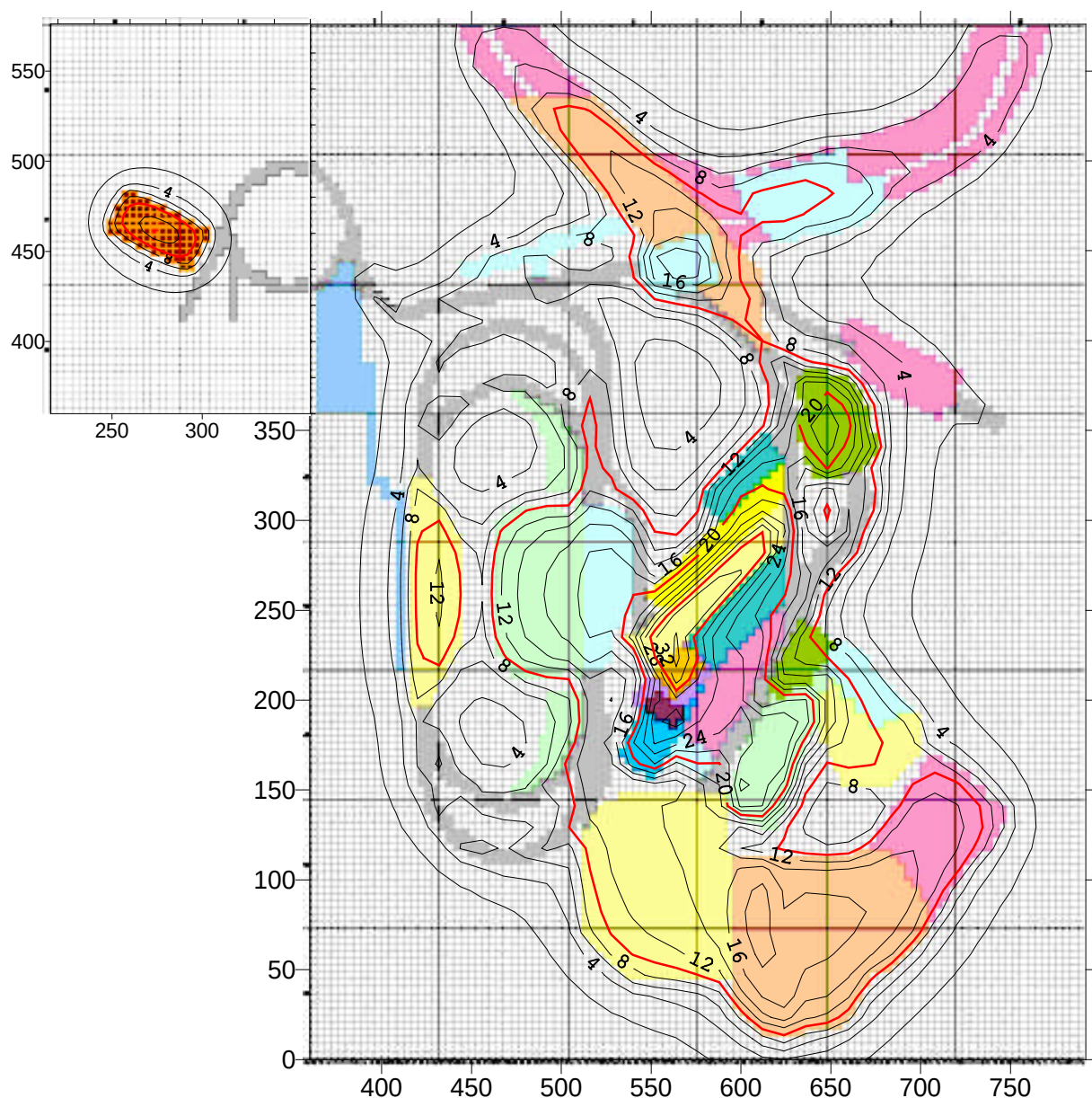
Bild 7.2: Setzungen aus Gebäudelasten
