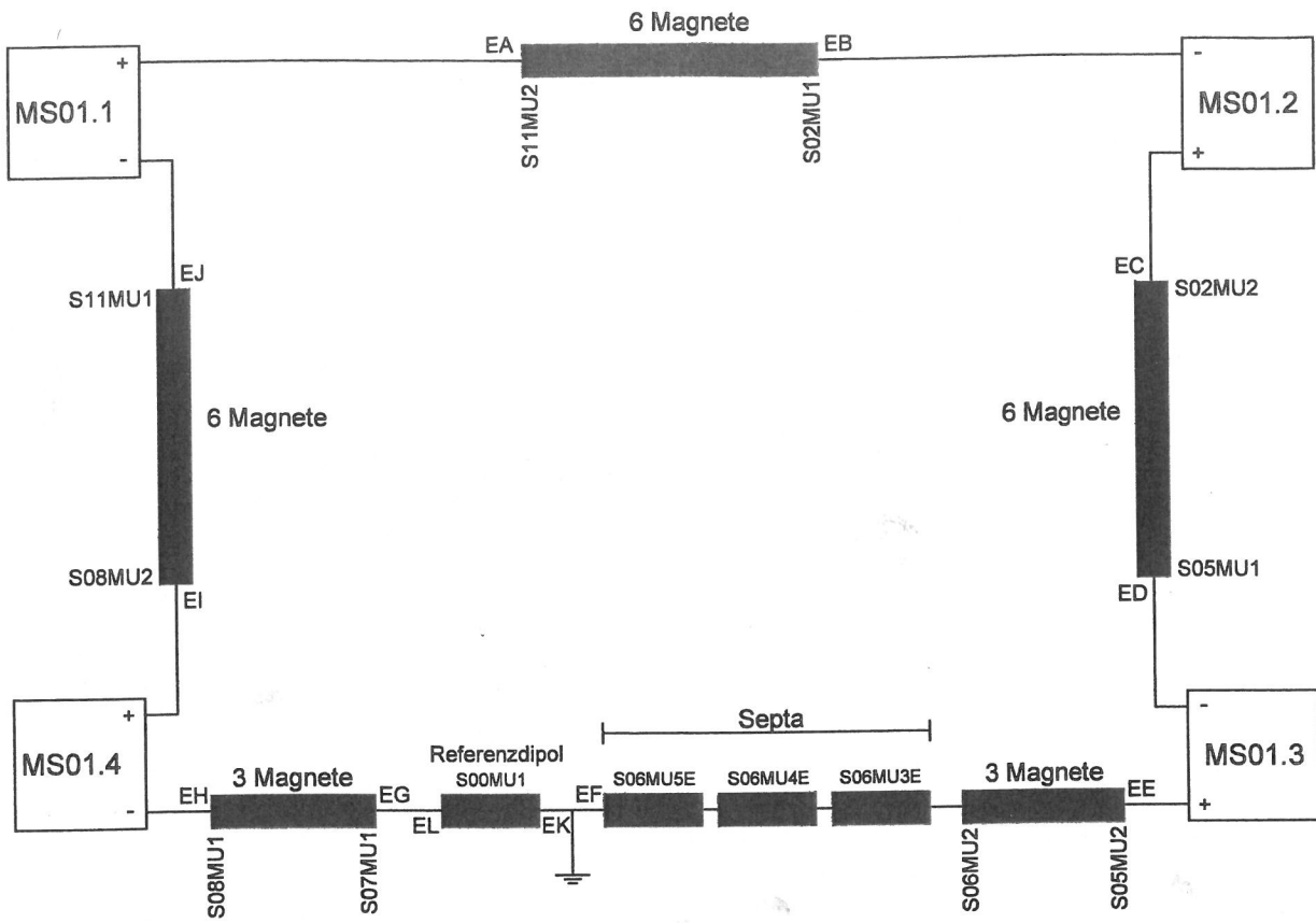
Schaltung für SIS-12 Betrieb
