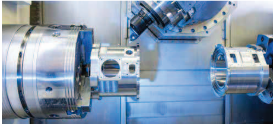
Drehen und Fräsen auf einer Maschine als 6-Seiten-Komplettbearbeitung: Dieses CNC-Bearbeitungszentrum verfügt über eine Haupt- und Gegenspindel für die wirtschaftliche Fertigung von Präzisionsbauteilen.
