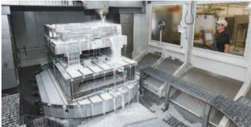
CNC-Fräsen eines großen, kubischen Werkstücks aus hochfester Aluminiumlegierung.
