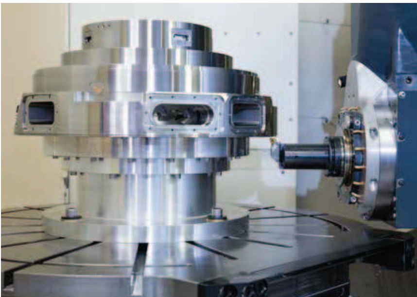
Dieses Fräs-/Drehzentrum mit planliegendem Maschinentisch bietet in einer Aufspannung alle Möglichkeiten der Zerspanung (bis \varnothing 1.250 mm). Die Werkstücke werden präzise ausgerichtet und wie auf einer Karusselldrehmaschine bearbeitet. Zusätzlich können sie 5-achsig gefräst sowie direkt auf der Maschine mit höchster Genauigkeit zu komplexen Baugruppen montiert werden.
